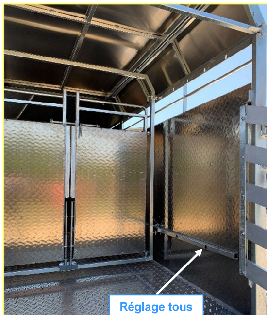
Séparation intérieure 2 battants sur rail
